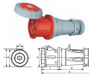
IP67 CEE/IEC 连接器 125A
