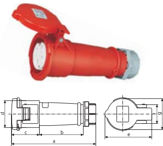
IP44 CEE/IEC 连接器 32A
