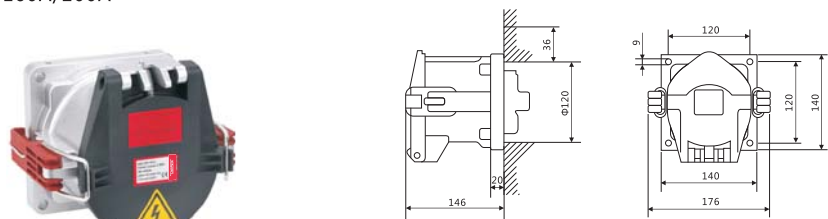
(外形尺寸图200A)
