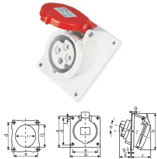
IP44 CEE/IEC 暗装斜插座 16A
