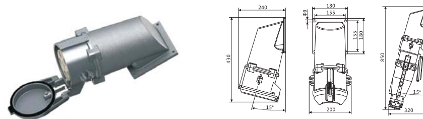
明装插座 250A/400A
