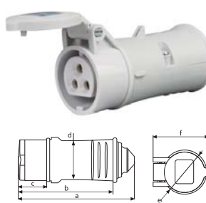
IP44 CEE/IEC 低压连接器 32A
