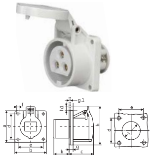
IP44 CEE/IEC 低压插座 16A
