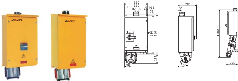
明装插座箱 160A/200A
