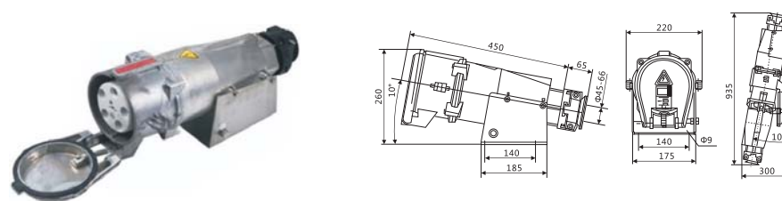
明装插座 250A/400A
