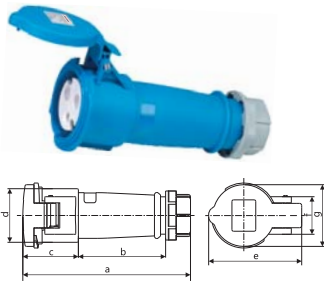
IP44 CEE/IEC 连接器 16A
