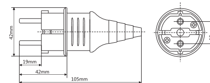
IP54 CEE/IEC Schuko 插头(ZH10838)
