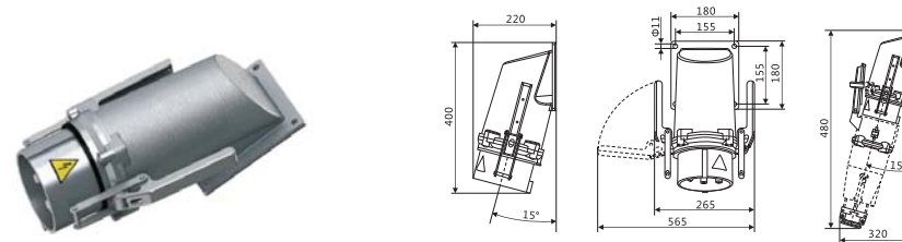
明装插头 250A/400A
