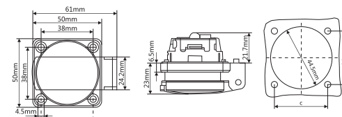
IP54 CEE/IEC Schuko 插座(ZH11031)
