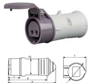
IP44 CEE/IEC 低压连接器 16A
