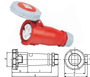
IP67 CEE/IEC 连接器 16A
