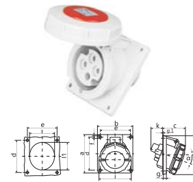
IP67 CEE/IEC 暗装斜插座 32A
