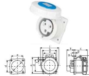
IP67 CEE/IEC 暗装直插座 16A
