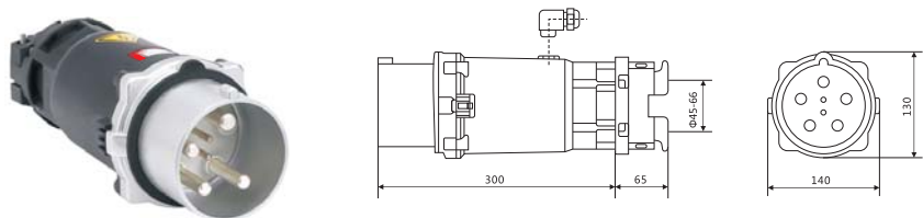
(外形尺寸图200A)
