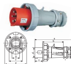
IP67 CEE/IEC 插头 125A
