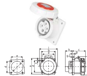
IP67 CEE/IEC 暗装直插座 32A
