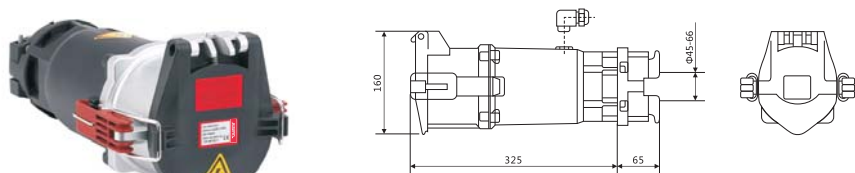
(外形尺寸图200A)
