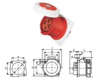
IP67 CEE/IEC 暗装直插座 125A
