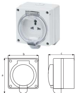
IP55多用插座
