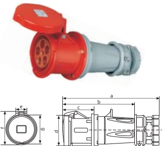
IP44 CEE/IEC 连接器 63A
