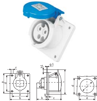
IP44 CEE/IEC 暗装直插座 16A
