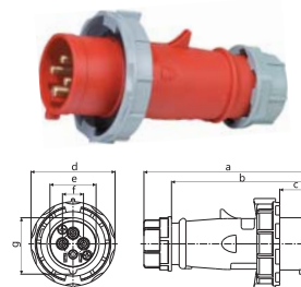
IP67 CEE/IEC 插头 32A
