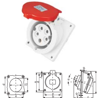
IP44 CEE/IEC 暗装斜插座 32A
