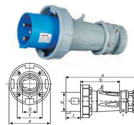
IP67 CEE/IEC 插头 63A
