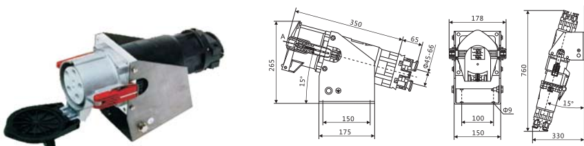
明装插座 160A/200A
