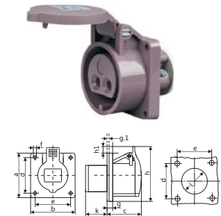
IP44 CEE/IEC 低压插座 32A
