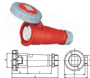
IP67 CEE/IEC 连接器 32A
