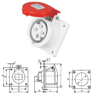
IP44 CEE/IEC 暗装直插座 32A
