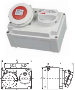
IP67 CEE/IEC 机械联锁 16A
