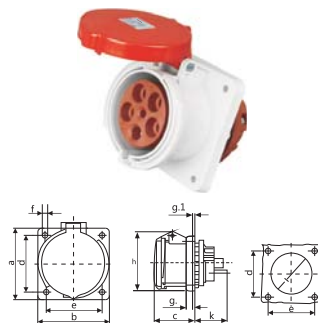
IP44 CEE/IEC 暗装直插座 63A
