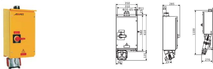
明装插座箱 160A/200A
