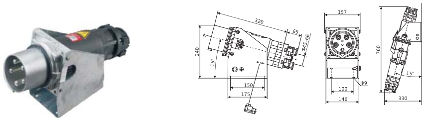
明装插头 160A/200A
