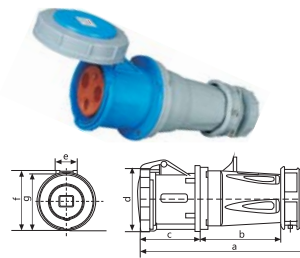
IP67 CEE/IEC 连接器 63A
