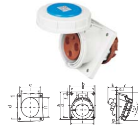
IP67 CEE/IEC 暗装斜插座 63A
