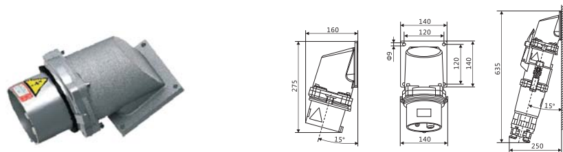
明装插头 160A/200A
