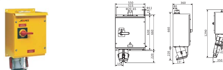
明装插座箱 250A/400A
