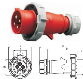
IP67 CEE/IEC 插头 16A
