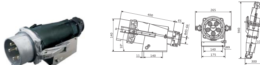
明装插头 250A/400A
