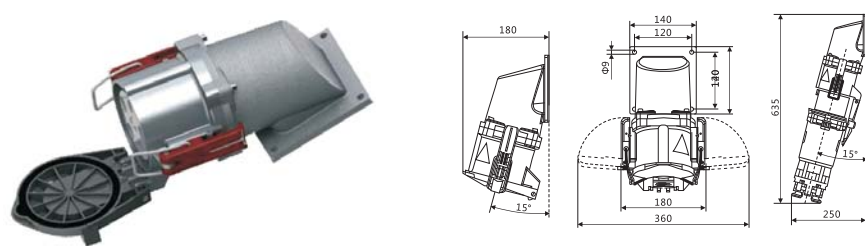
明装插座 160A/200A
