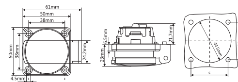
IP54 CEE/IEC 多功能暗装插座(ZH312D)
