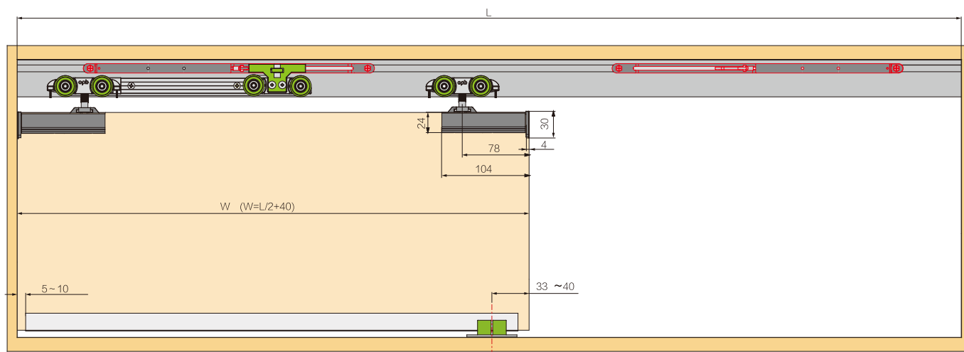
木门2 Wood Door 2
