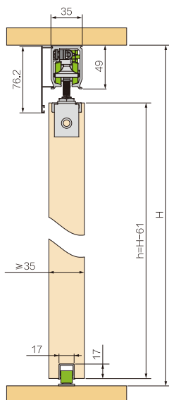
木门1 Wood Door 1
