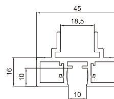
XNA162 上下横 Upper&bottom frame
