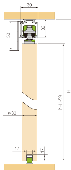
木门3 Wood Door 3
