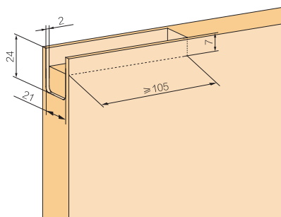
门板开槽尺寸 Door Panel Grooving Size
