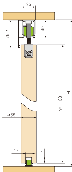
木门2 Wood Door 2
