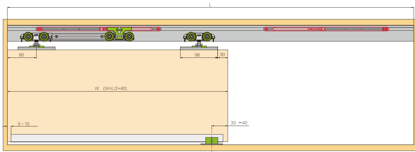
木门3 Wood Door 3
