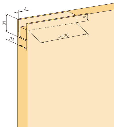
门板开槽尺寸 Door Panel Grooving Size
