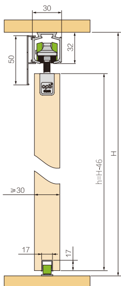
木门2 Wood Door 2
