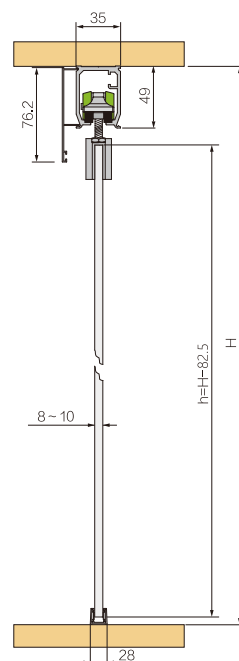
玻璃门5 Glass Door 5
