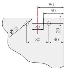
玻璃开孔尺寸 Glass Hole Size
