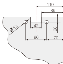
玻璃开孔尺寸 Glass Hole Size
