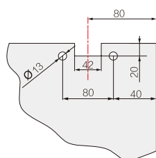
玻璃开孔尺寸 Glass Hole Size
