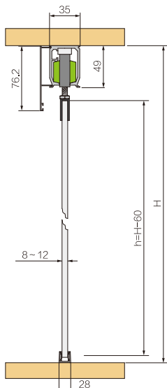
玻璃门4 Glass Door 4
