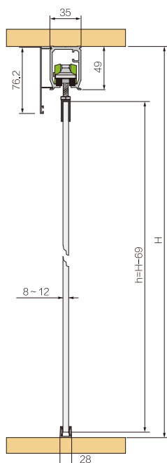
玻璃门4 Glass Door 4
