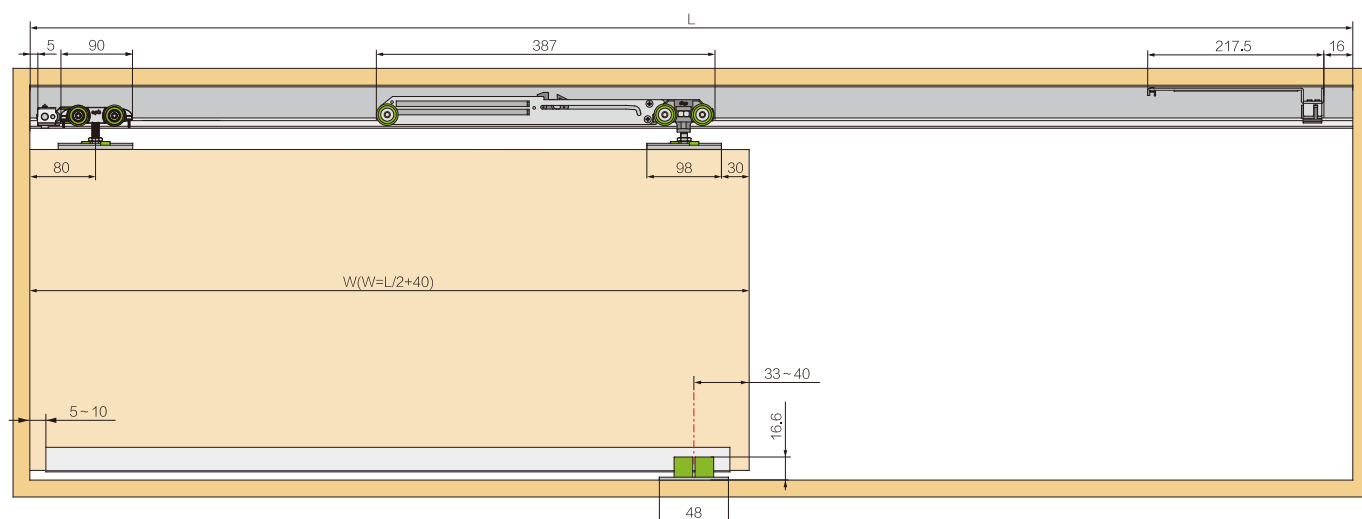
木门3 Wood Door 3
