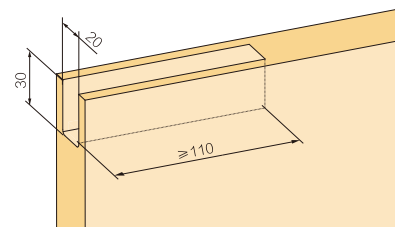
门板开槽尺寸 Door Panel Grooving Size
