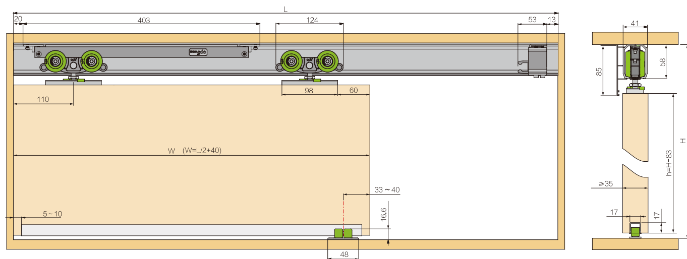
门板开槽尺寸 Door Panel Grooving Size
