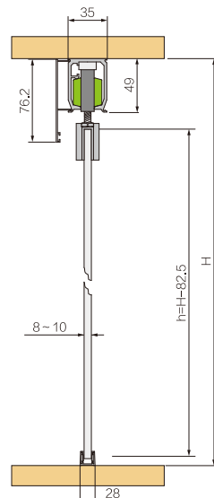
玻璃门5 Glass Door 5
