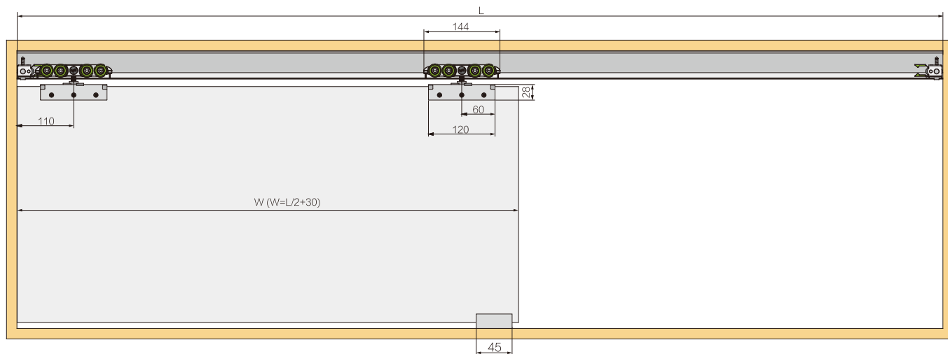
玻璃门5 Glass Door 5
