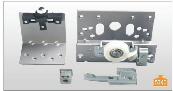
OPK-30144 Top Hang System-Outer Door
