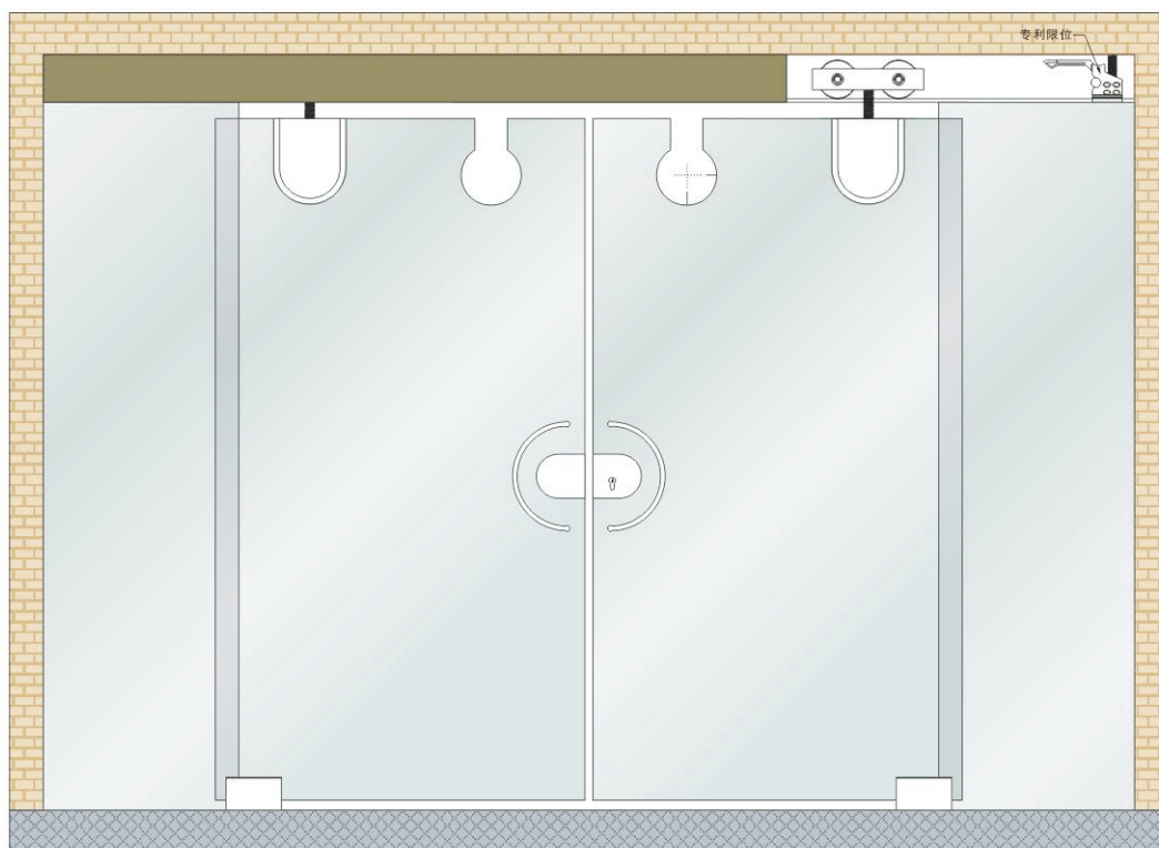
OPK-3-8K Sliding Glass Door Roller Fitting
