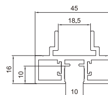
XNA162 上下横 Upper&bottom frame
