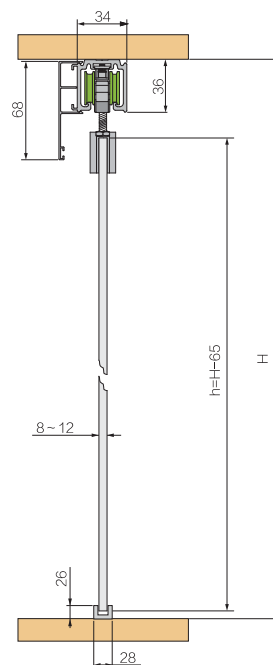
玻璃门5 Glass Door 5
