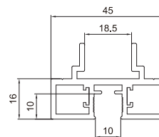
XNA162 上下横 Upper&bottom frame
