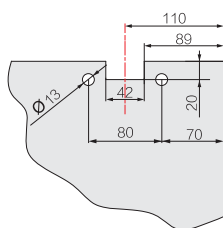
玻璃开孔尺寸 Glass Hole Size
