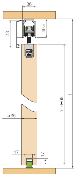
木门2 Wood Door 2
