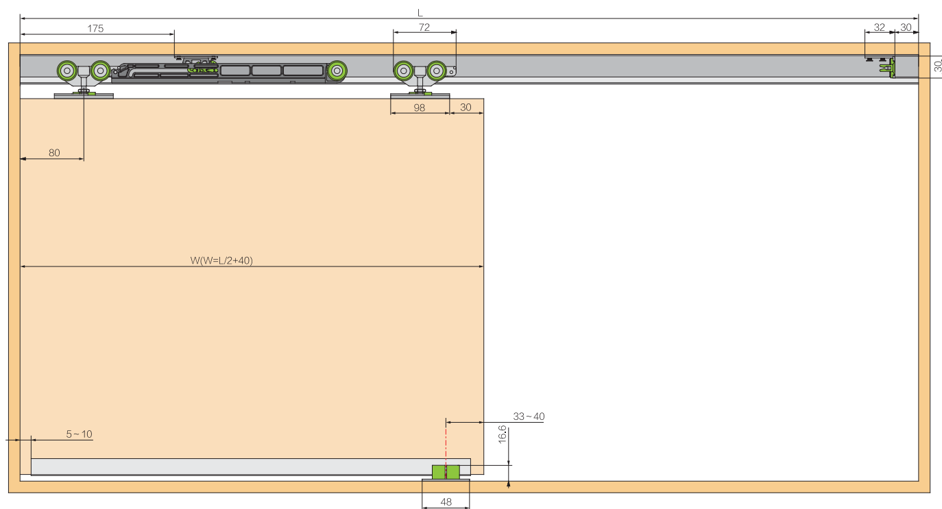
木门3 Wood Door 3
