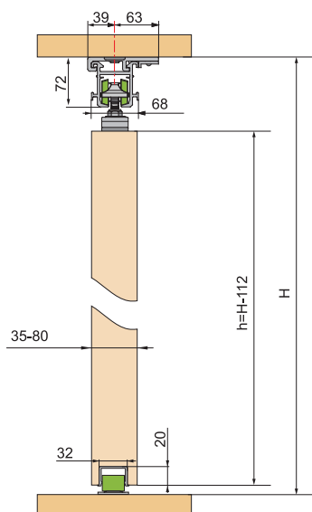
无阻尼 Without Damping
