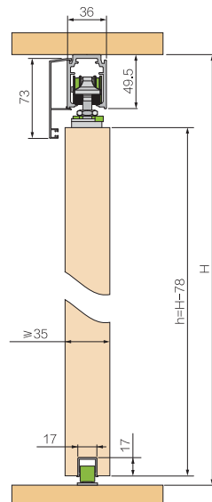
木门3 Wood Door 3
