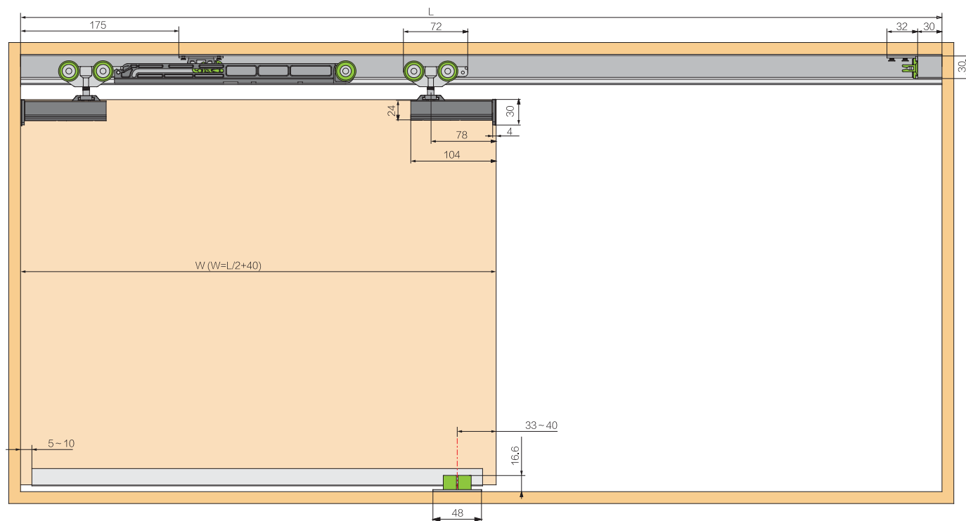
木门2 Wood Door 2
