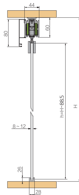
玻璃门5 Glass Door 5
