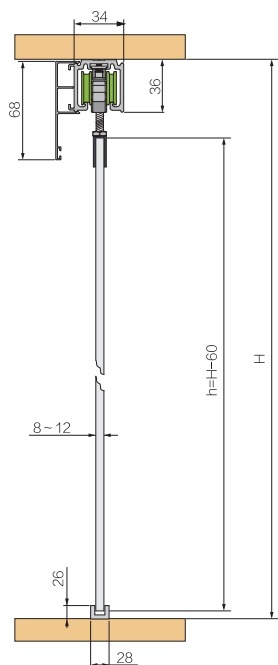
玻璃门4 Glass Door 4
